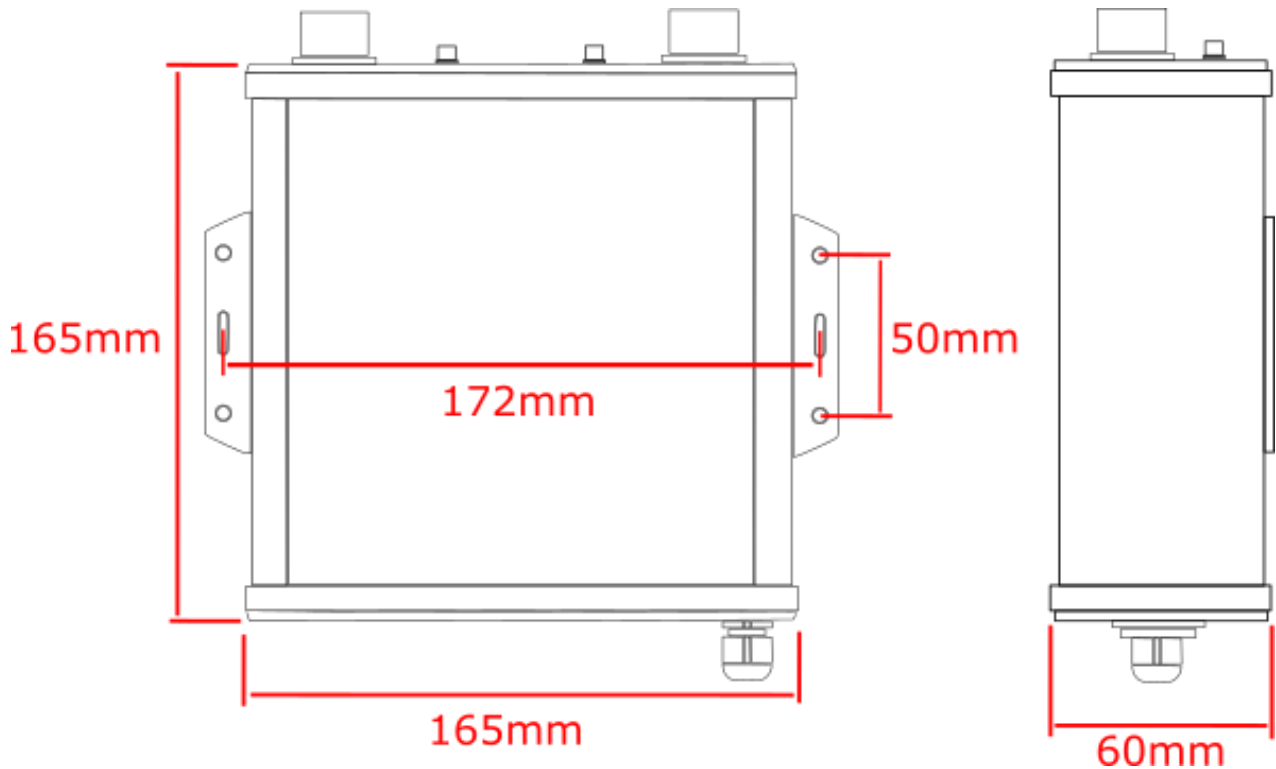
Abbildung 1 - Abmessungen
