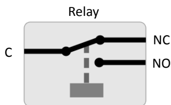
Funzionamento interno del relè programmabile
