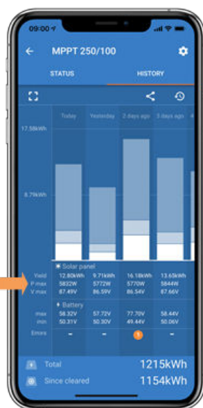
Cronologia della Pmax in VictronConnect
