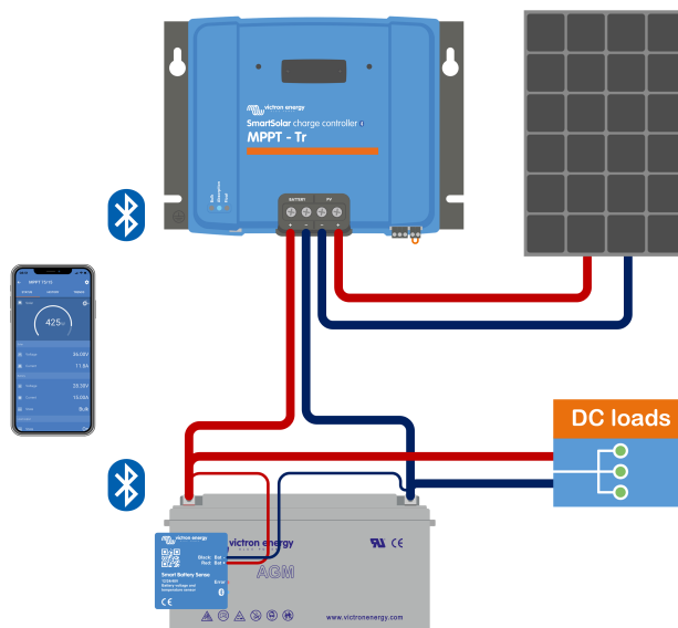
Esempio di Rete VE.Smart di un Rilevatore Smart Battery e un caricabatterie solare
