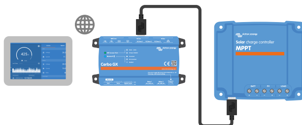
Connessione App VictronConnect tramite LAN o internet (portale VRM) e un dispositivo GX (ad esempio, un Cerbo GX)
