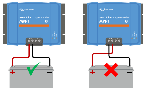
Esempi di polarità corretta ed erronea (inversa) della batteria
