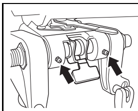
Drehgelenkkonsole
